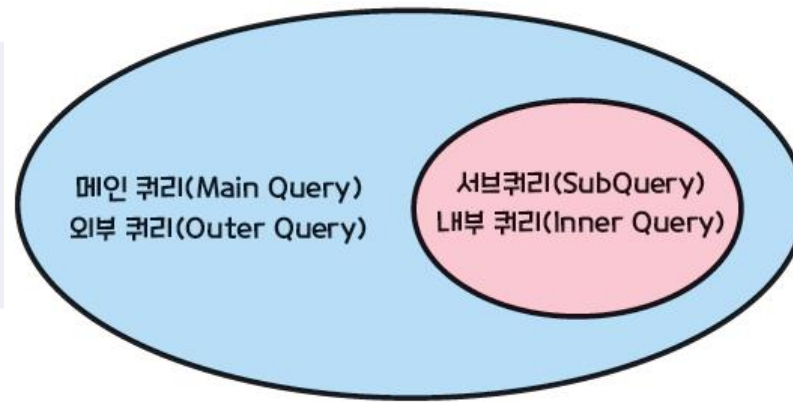
서브쿼리의 구조
